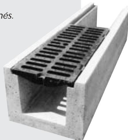
Caniveau à feuillure béton avec grille
