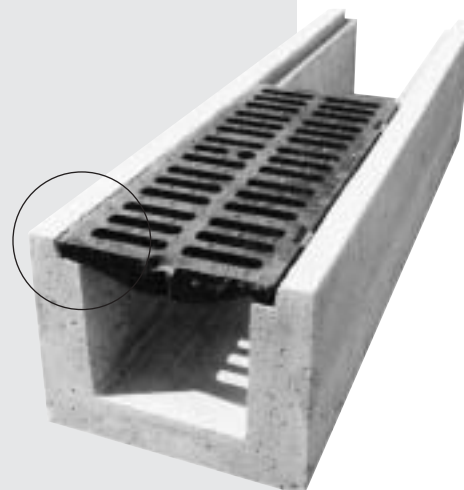
Caniveau avec cornière
